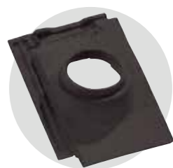
Tuile à douille BEAUVOISE Graphite Ø 126 (conforme VMC) Réf. 312.31
