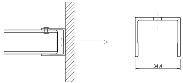
Profilé U
