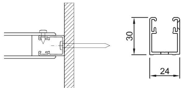
Profilé en joint-croix (option)
