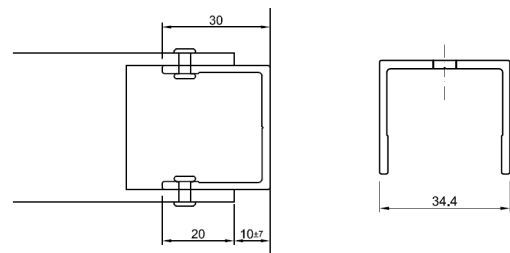
Profilé en joint-croix (option)
