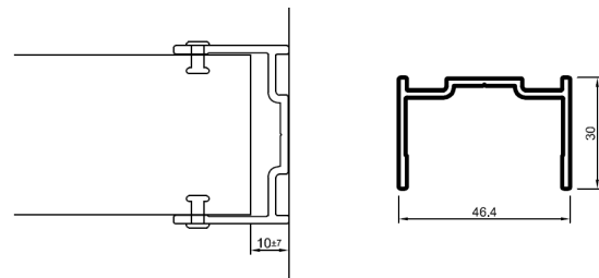
Profilé U
