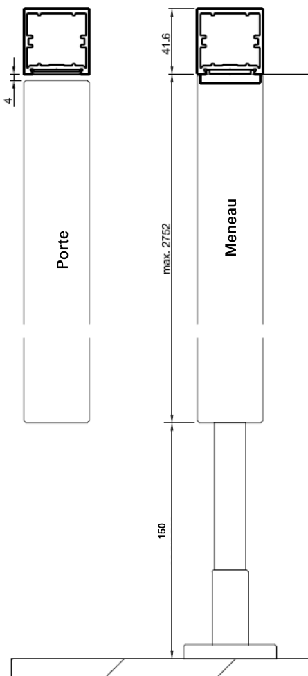
Coupe configuration standard
