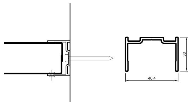
Profilé U
