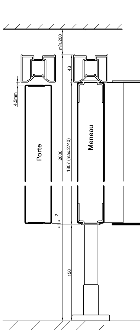
Coupe configuration standard
